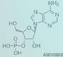
ADENOSINE
